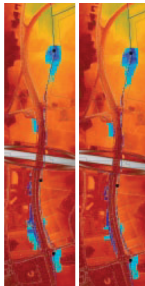
Figuur 11.5 Overstromingsrisico 1 x per 10 jaar in landelijk gebied huidige situatie (links) en plansituatie (rechts).
